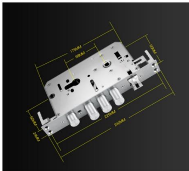
3) 九头霸王锁体
